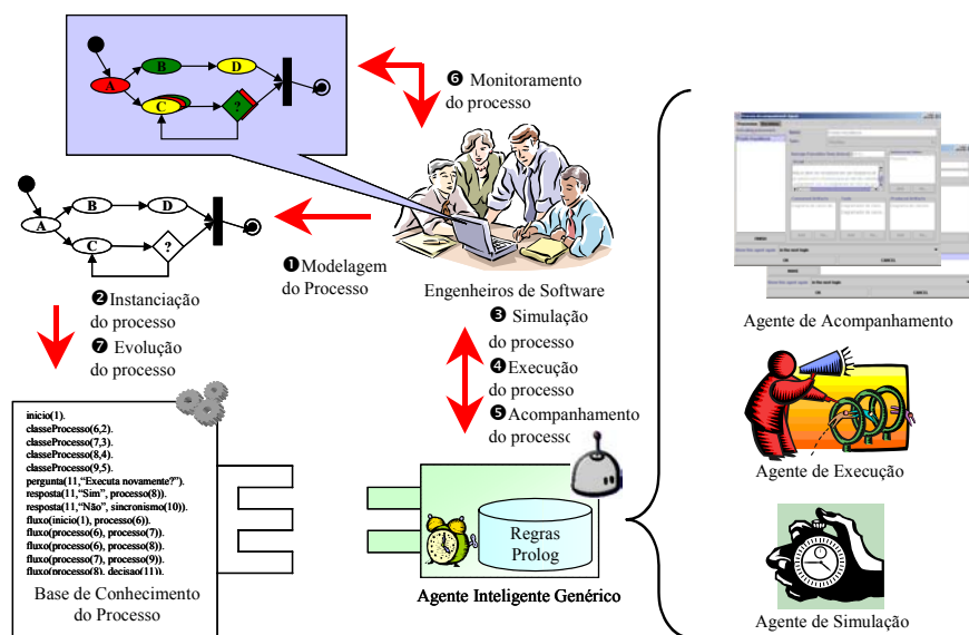
Figura 3.2: Atividades envolvidas na abordagem Charon.
