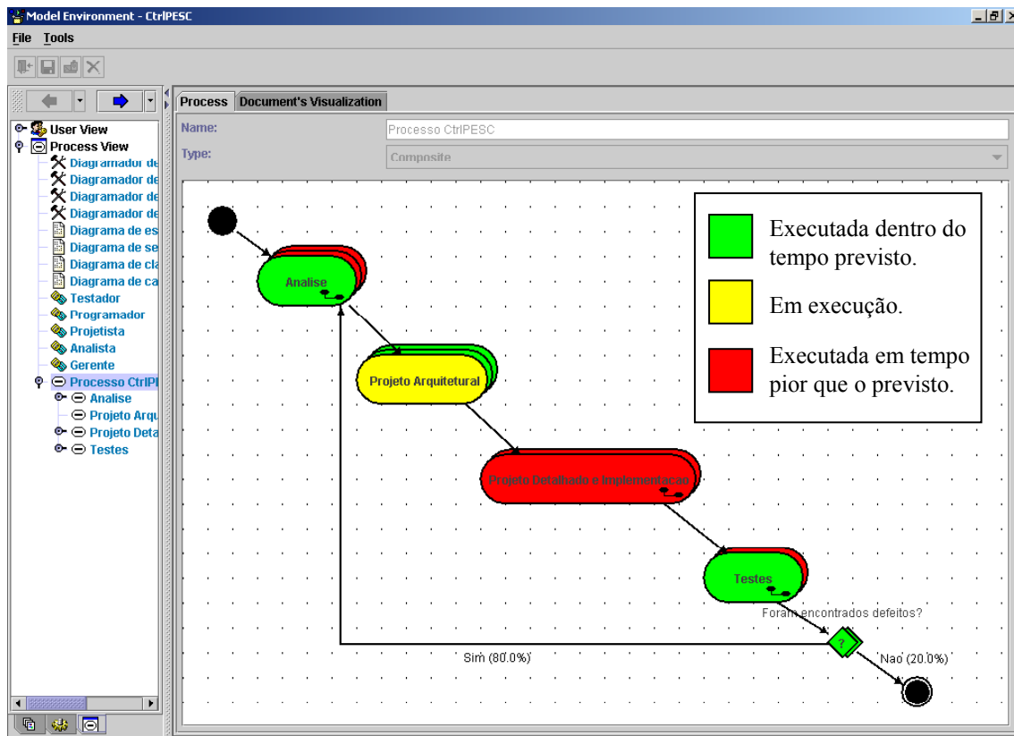
Figura 4.12: Monitoramento do processo principal.
