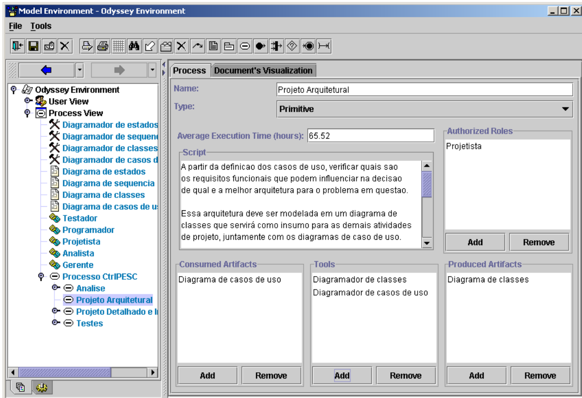
Figura 4.3: Modelagem do processo que representa a atividade de projeto detalhado.
