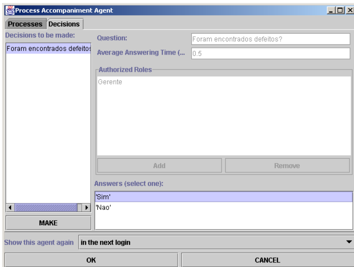
Figura 4.10: Finalização de decisão em execução.
