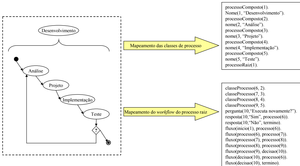
Figura 3.8: Exemplo do mapeamento de processos segundo a ontologia proposta.
