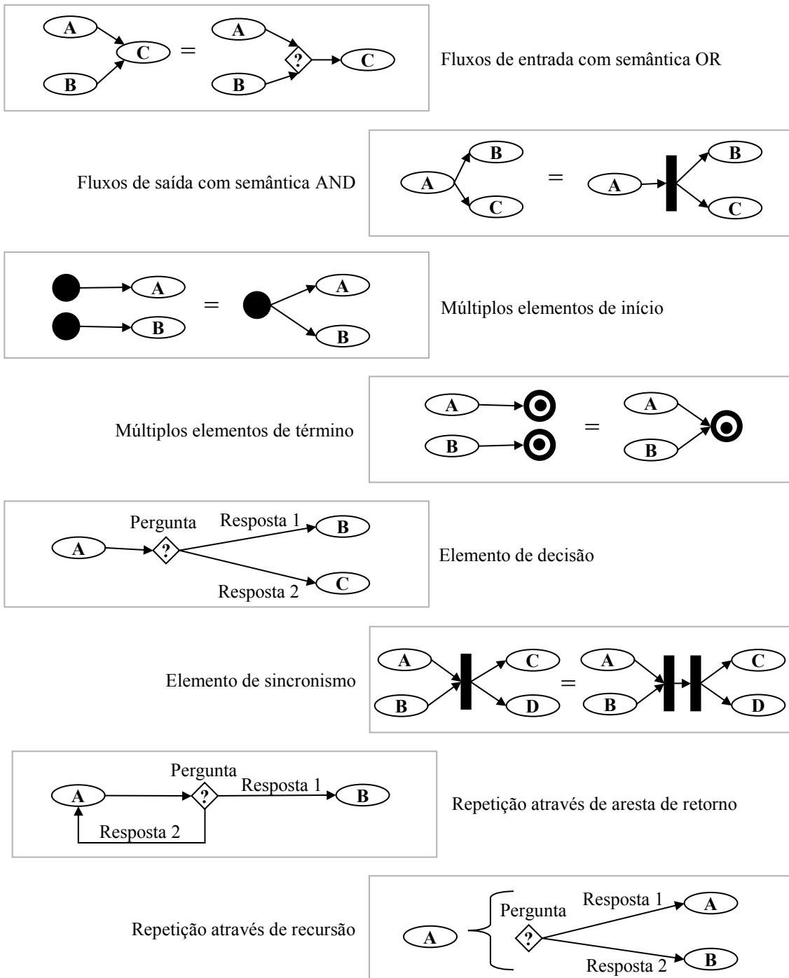
Figura 3.5: Notação do diagrama de atividades UML estendido.
