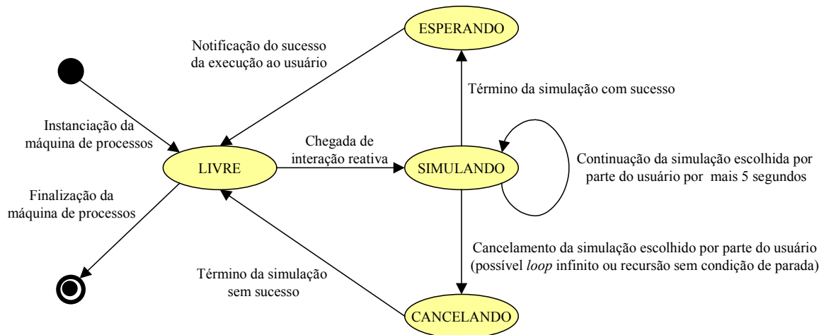
Figura 3.11: Diagrama de transição de estados do Agente de Simulação.
