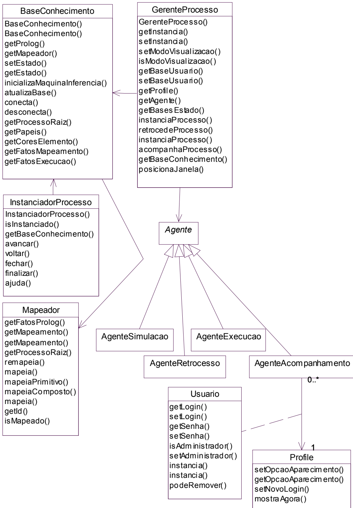
Figura 4.1: Detalhamento técnico do protótipo.
