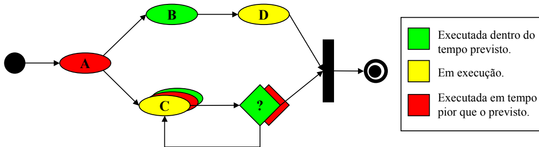
Figura 3.12: Exemplo da notação de monitoramento da execução de processos.
