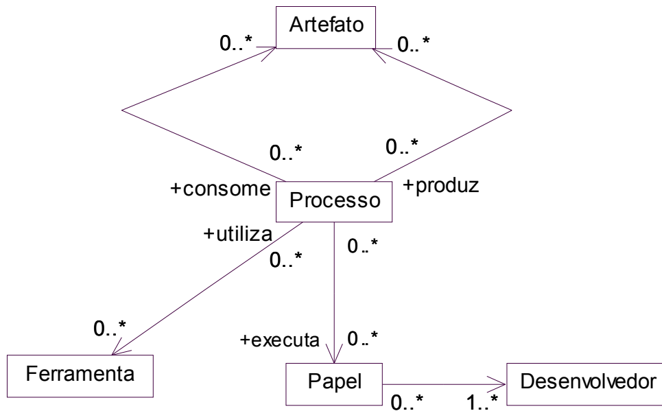
Figura 3.3: Modelo de processo primitivo utilizado pela abordagem proposta.
