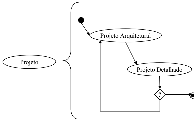
Figura 3.6: Repetição da execução através de fluxo de retorno.
