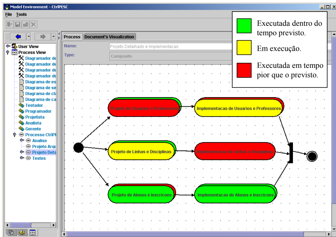
Figura 4.11: Monitoramento do processo de projeto detalhado e implementação.
