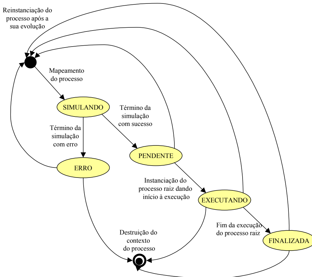
Figura 3.10: Diagrama de transição de estados da base de conhecimento.
