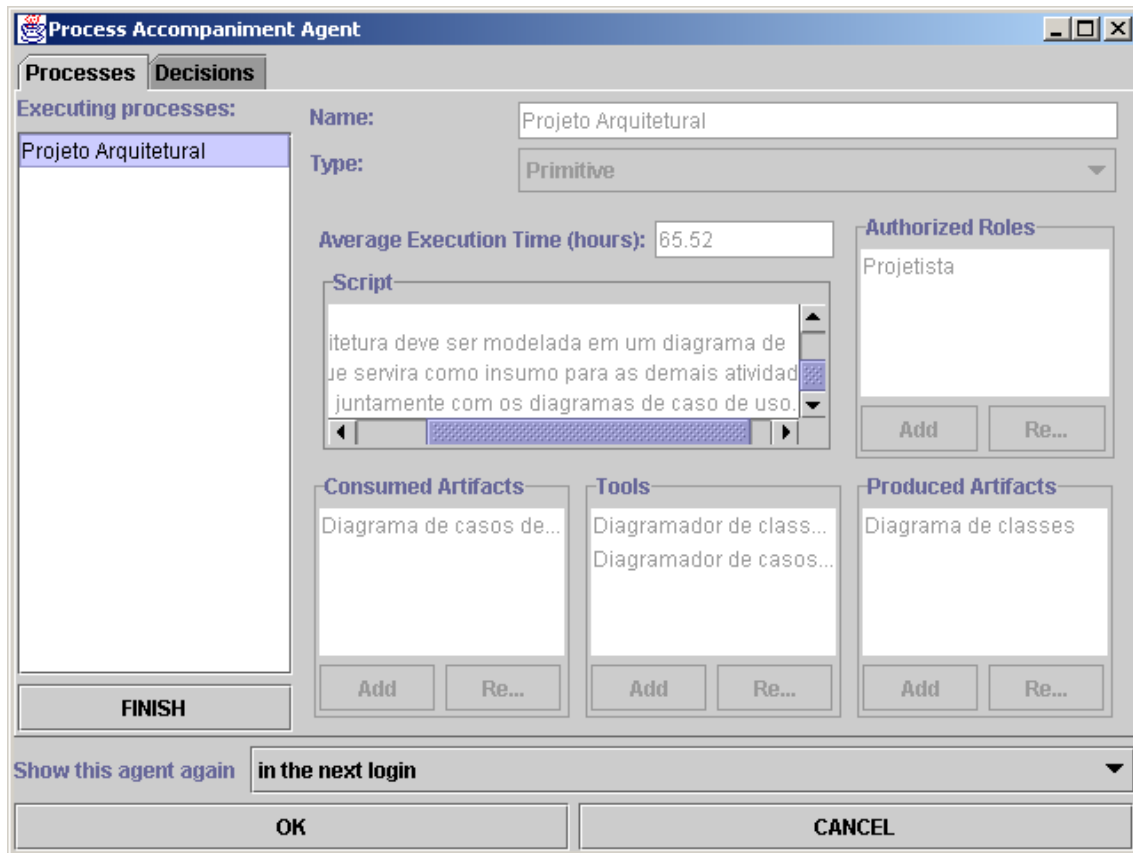
Figura 4.9: Finalização de processo em execução.
