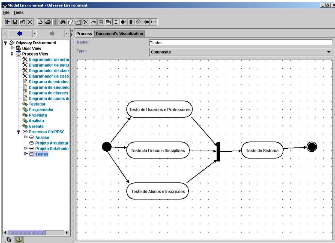
Figura 4.4: Modelagem do processo que representa a atividade de testes.
